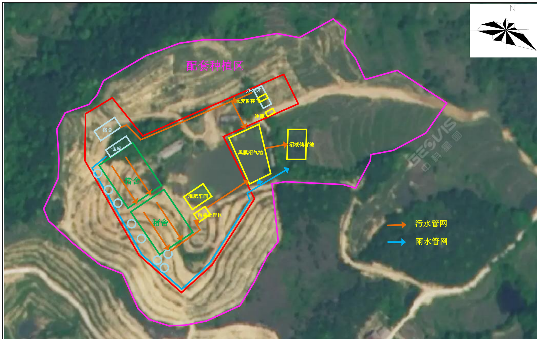
附图 7 项目雨污管网图
