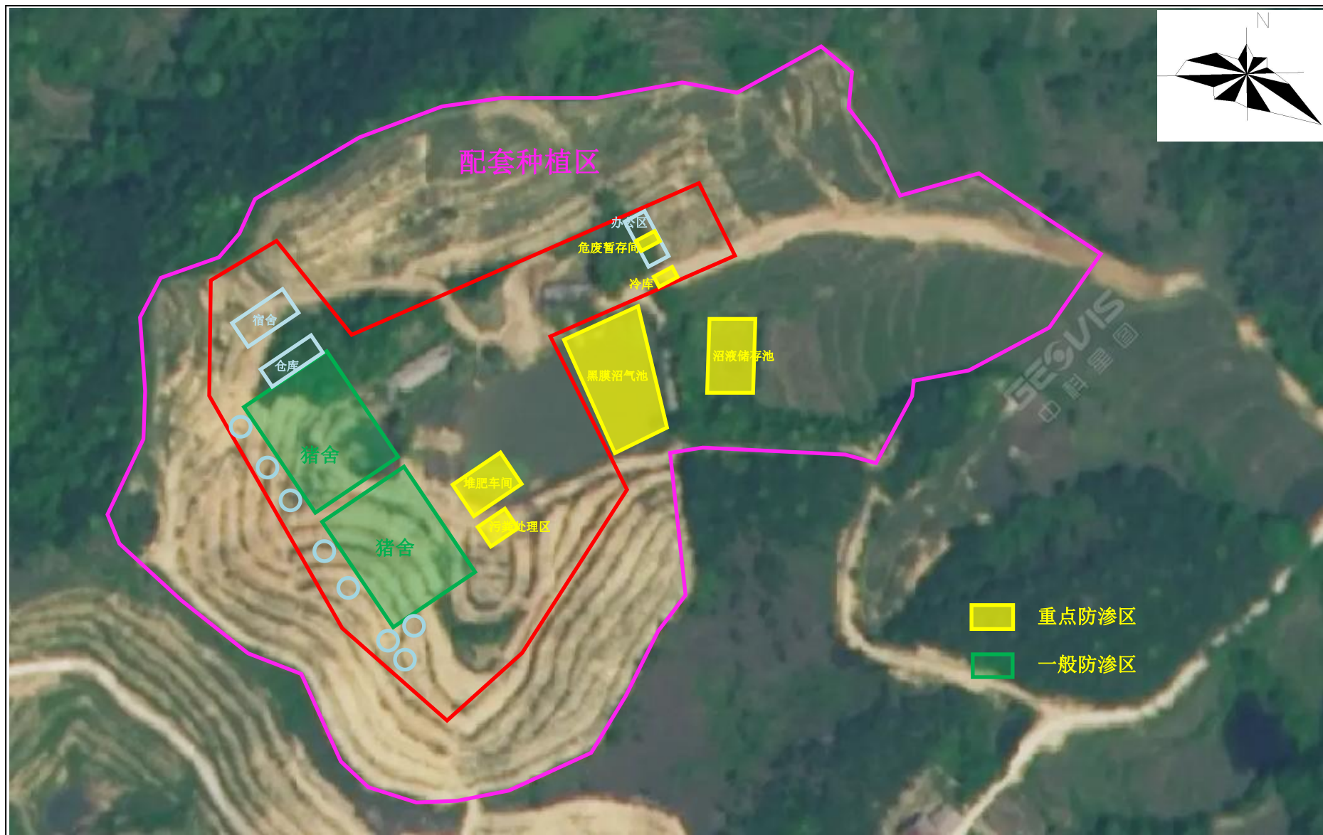
附图 6 项目分区防渗图
